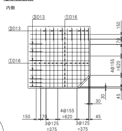
底板配筋図
