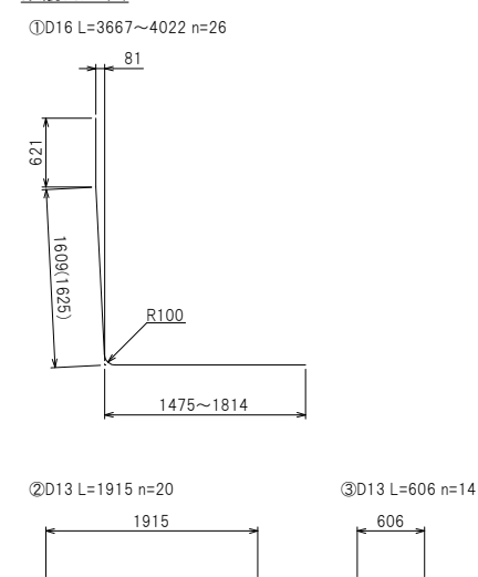
鉄筋加工図
