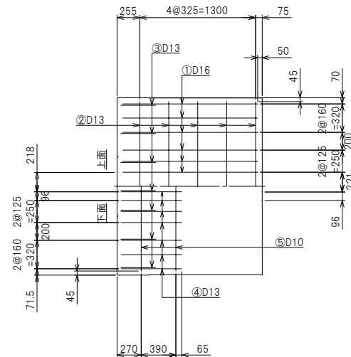
底板配筋図
