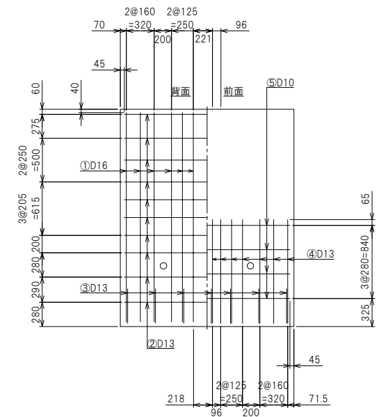
たて壁配筋図
