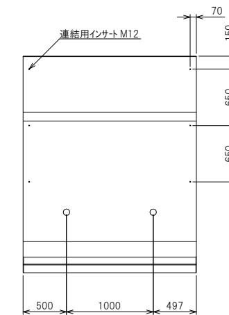
背面構造図
