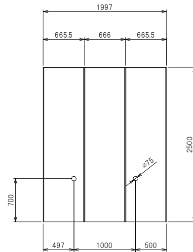
正面構造図
