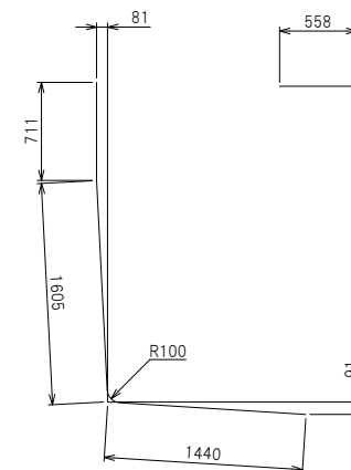
鉄筋加工図
