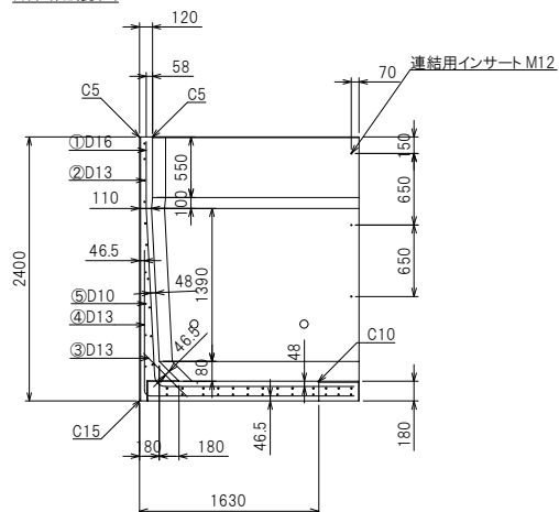
断面配筋図
