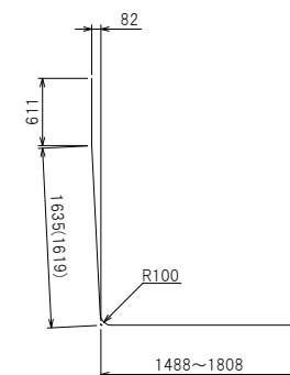
鉄筋加工図
