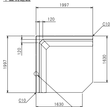
平面構造図
