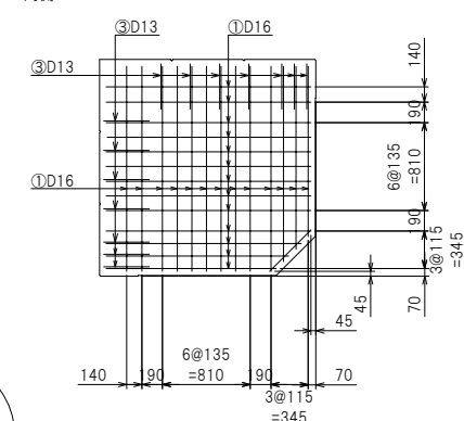
底版配筋図
