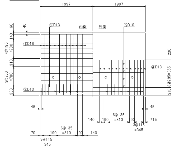
たて壁配筋図
