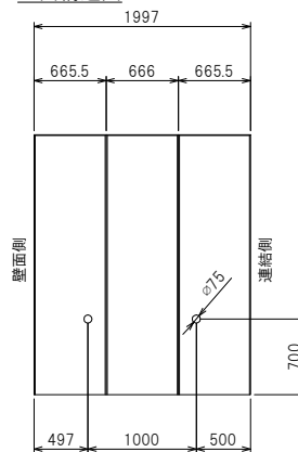
正面構造図
