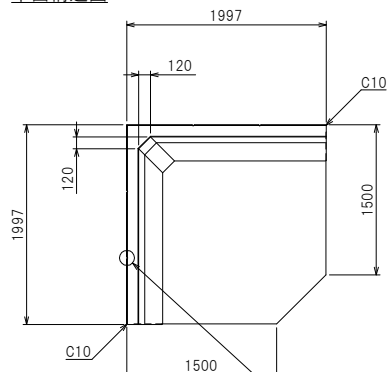
平面構造図
