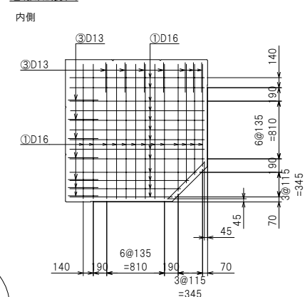
底板配筋図
