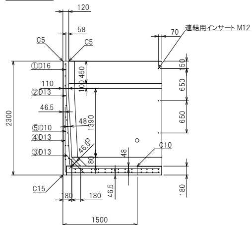
断面配筋図
