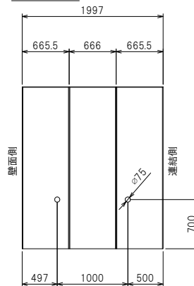
正面構造図
