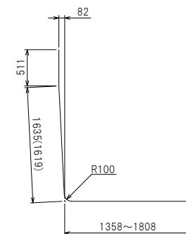
鉄筋加工図
