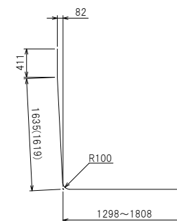
鉄筋加工図
