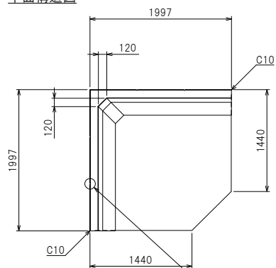
平面構造図
