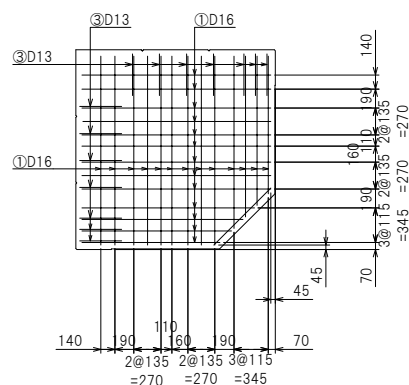
底版配筋図
