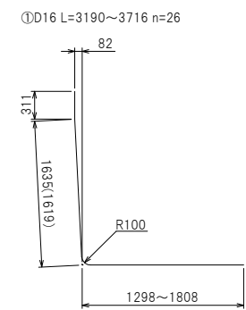
鉄筋加工図
