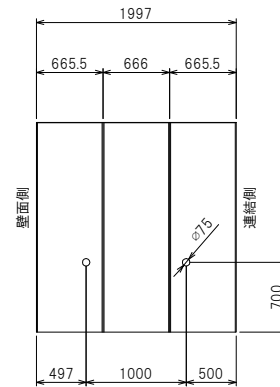
正面構造図
