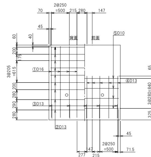
たて壁配筋図
