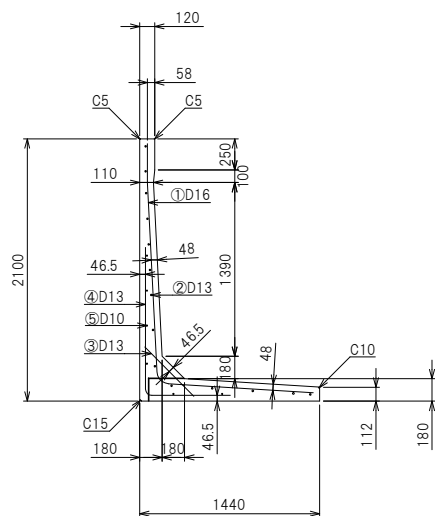
側面配筋図
