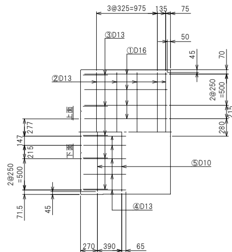
底板配筋図
