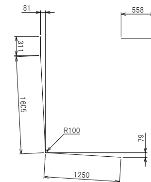
鉄筋加工図
