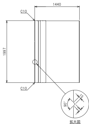
平面構造図
