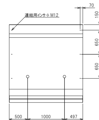
背面構造図
