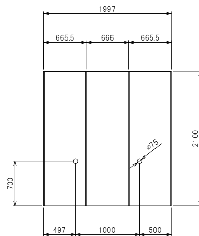
正面構造図
