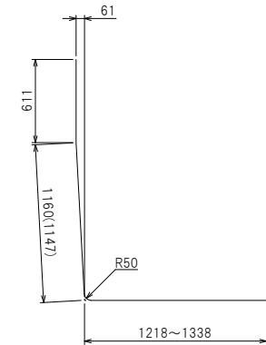
鉄筋加工図
