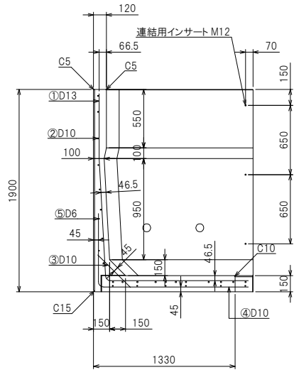
断面配筋図
