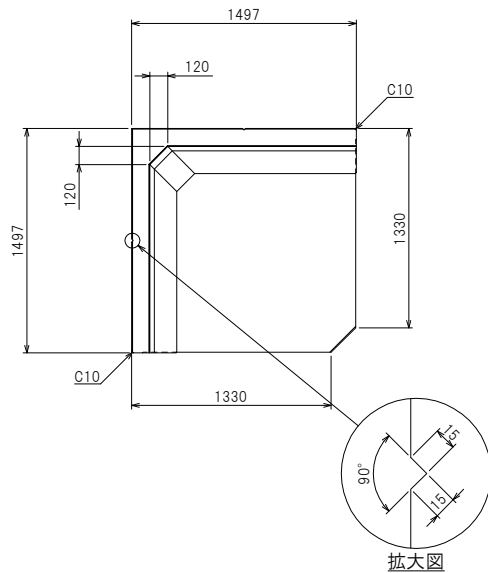
平面構造図
