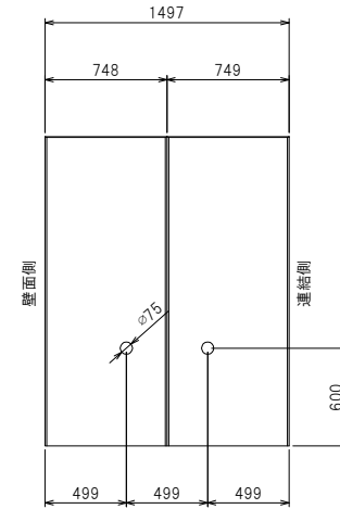
正面構造図
