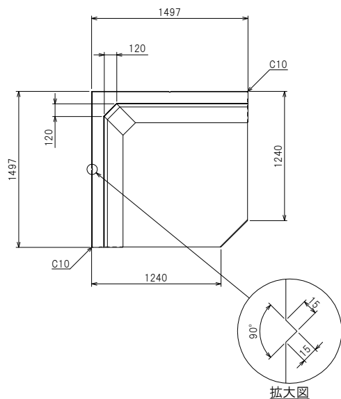
平面構造図
