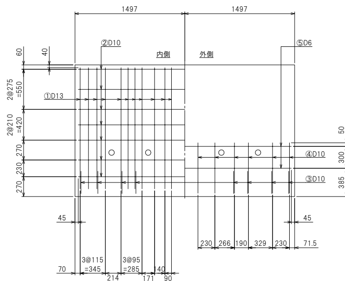
たて壁配筋図
