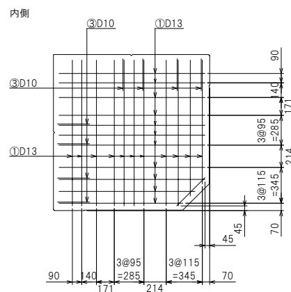
底板配筋図
