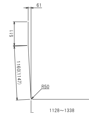
鉄筋加工図
