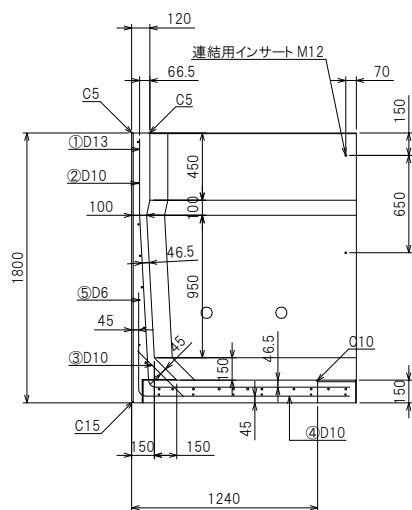
断面配筋図
