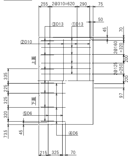
底板配筋図
