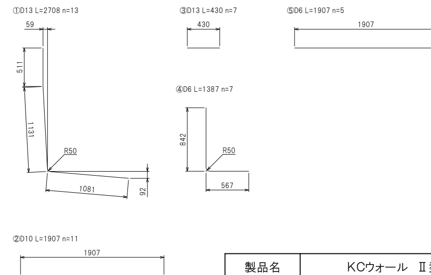
鉄筋加工図
