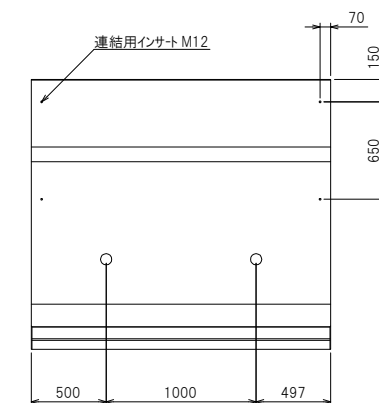
背面構造図
