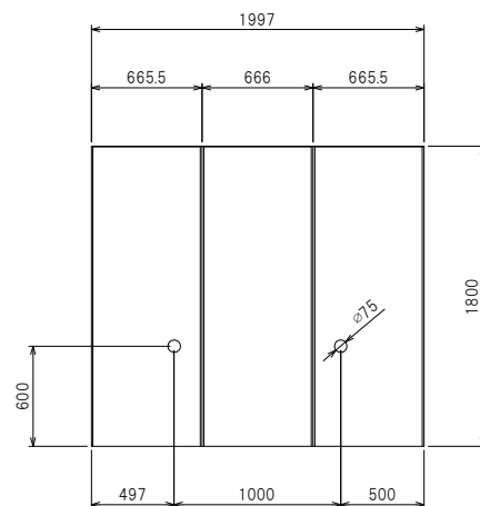
正面構造図
