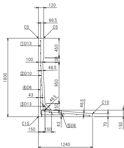
側面配筋図
