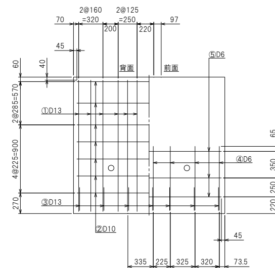
たて壁配筋図
