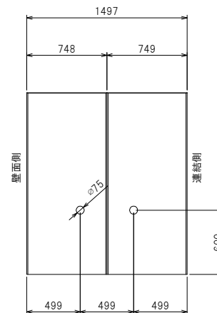
正面構造図
