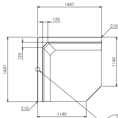
平面構造図
