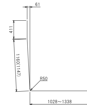
鉄筋加工図
