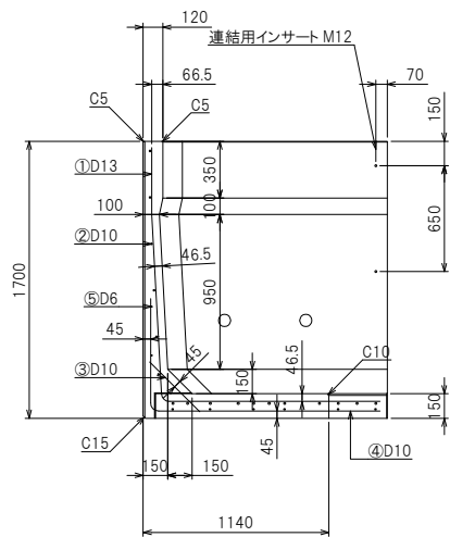
断面配筋図
