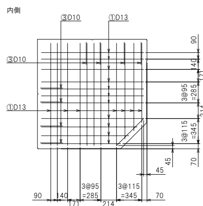
底板配筋図
