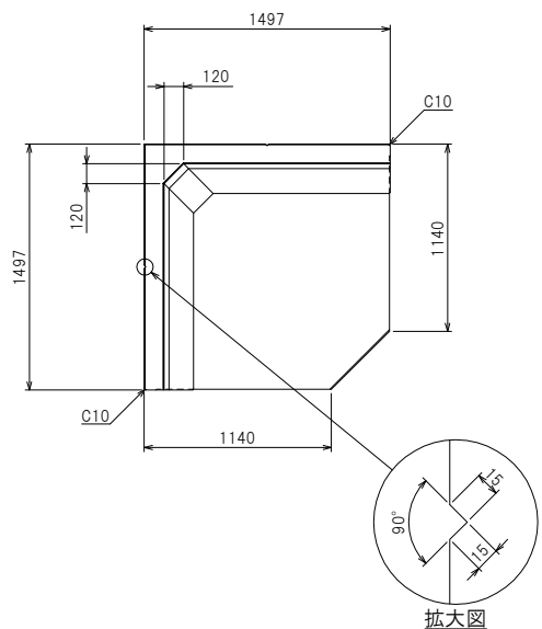
平面構造図
