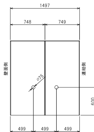
正面構造図
