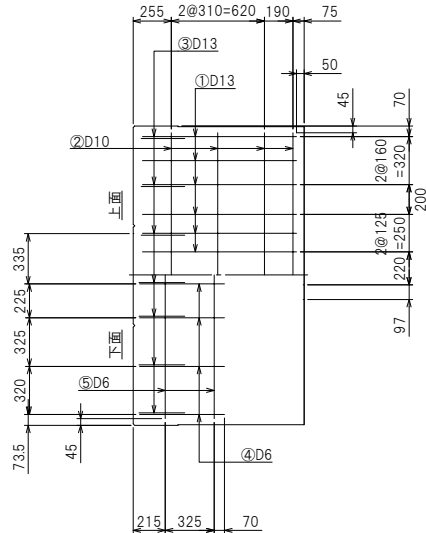
底板配筋図
