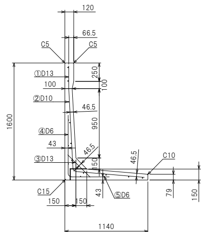
側面配筋図
