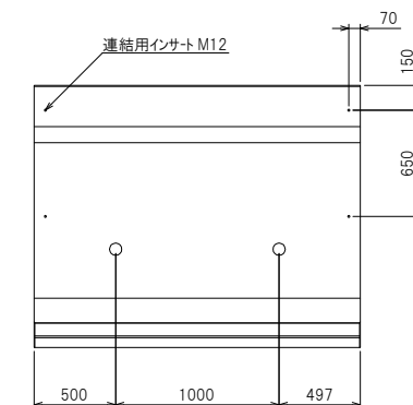
背面構造図
