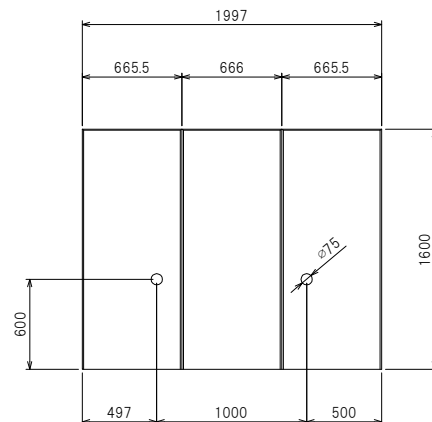
正面構造図
