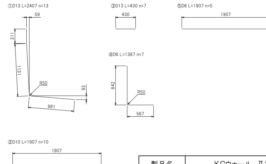
鉄筋加工図
