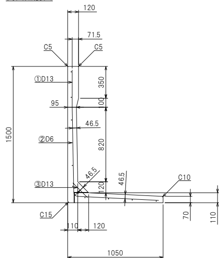
側面配筋図
