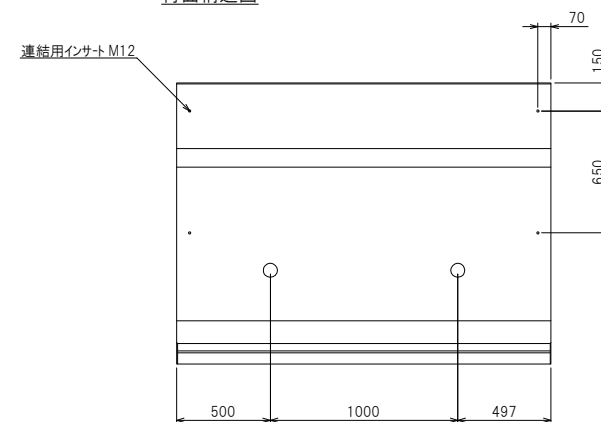
背面構造図
