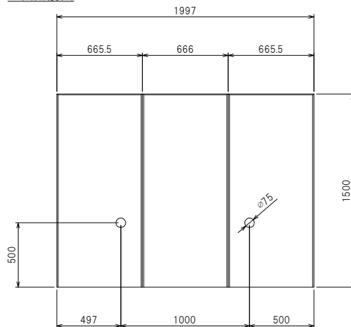
正面配筋図
