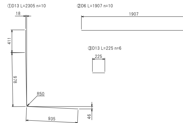
鉄筋加工図
