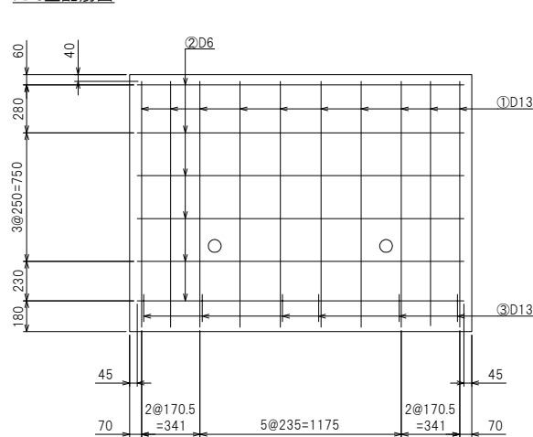
たて壁配筋図
