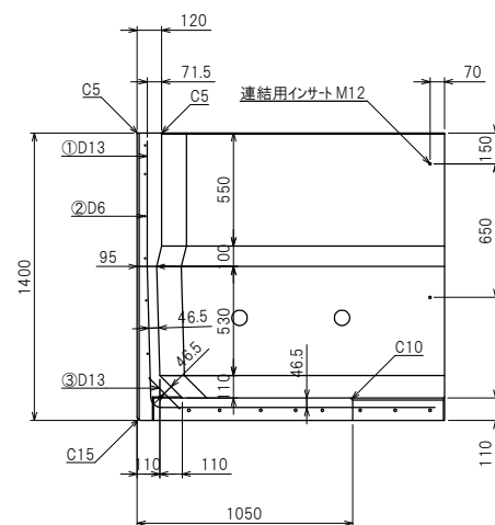
断面配筋図
