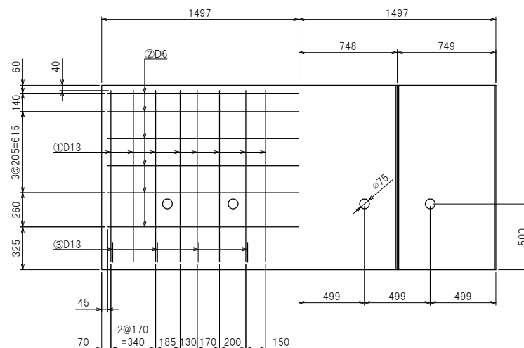
たて壁配筋図
