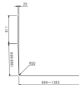
鉄筋加工図
