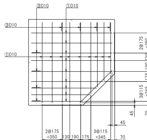
底版配筋図
