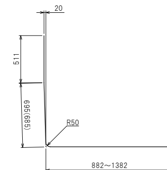
鉄筋加工図
