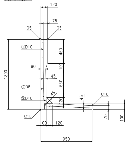
側面配筋図
