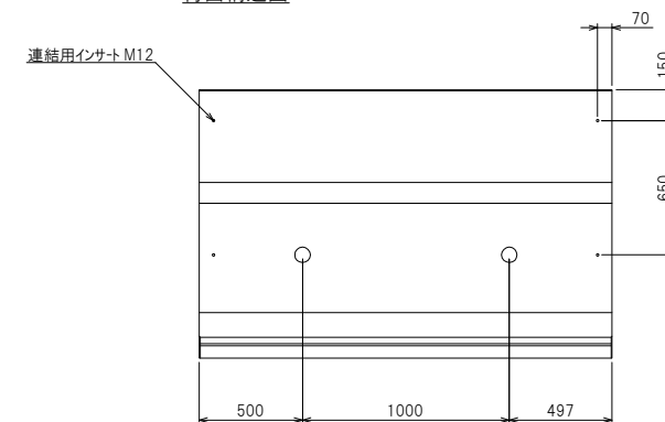
背面構造図
