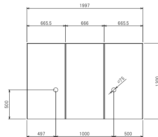
正面配筋図
