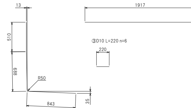
鉄筋加工図
