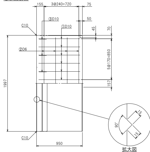
底板配筋図
