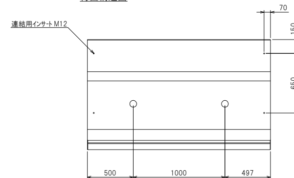
背面構造図
