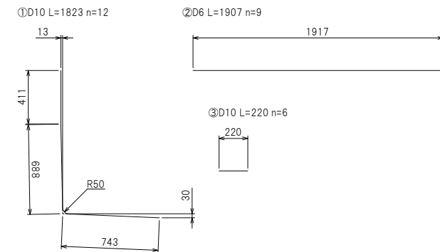
鉄筋加工図
