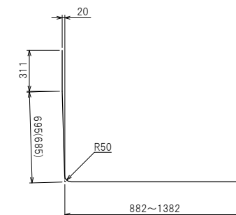
鉄筋加工図
