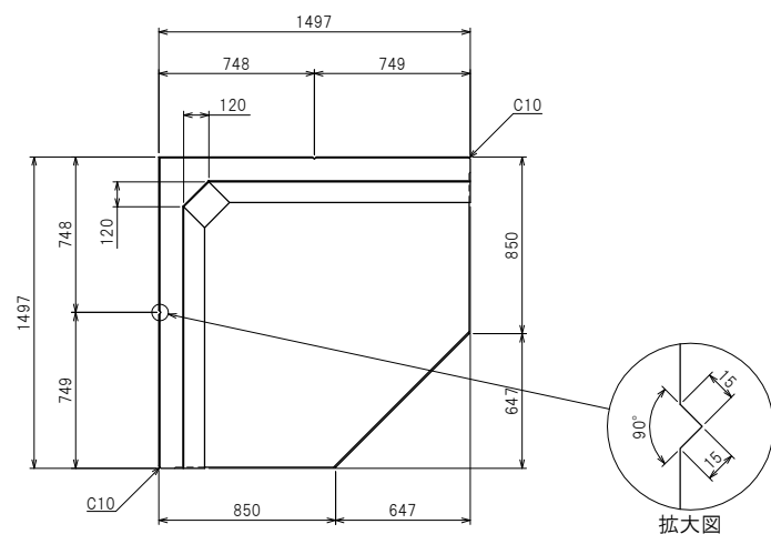
平面構造図
