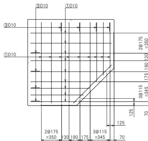
底板配筋図
