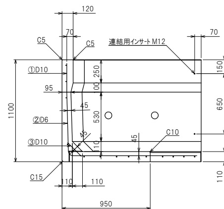
断面配筋図
