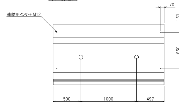
背面構造図
