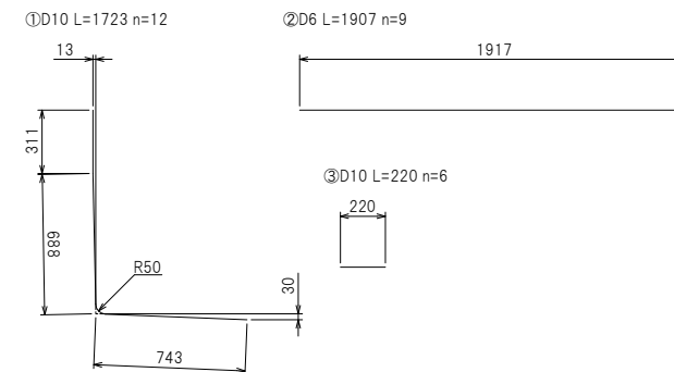
鉄筋加工図
