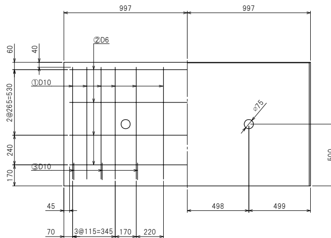
たて壁配筋図
