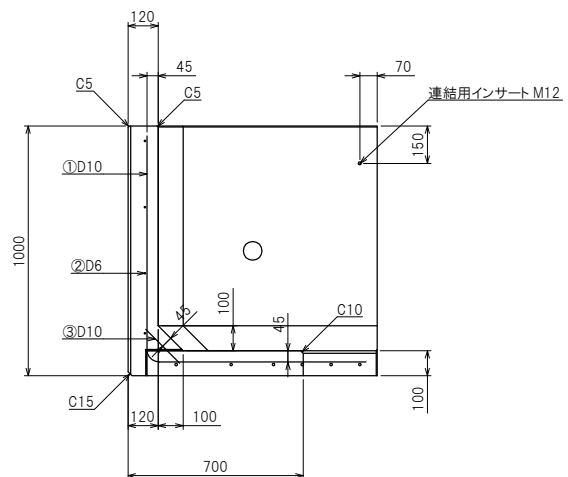
断面配筋図
