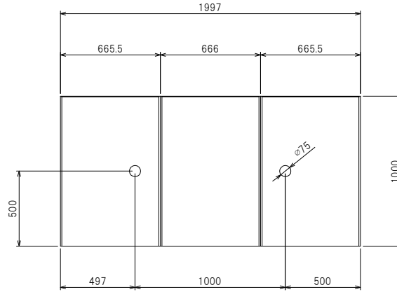
正面構造図
