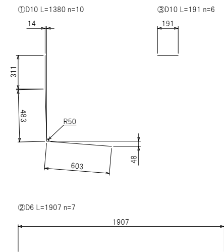
鉄筋加工図
