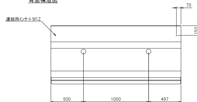
背面構造図
