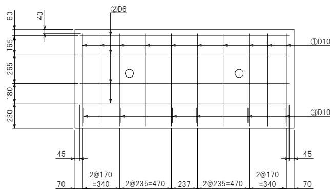
たて壁配筋図
