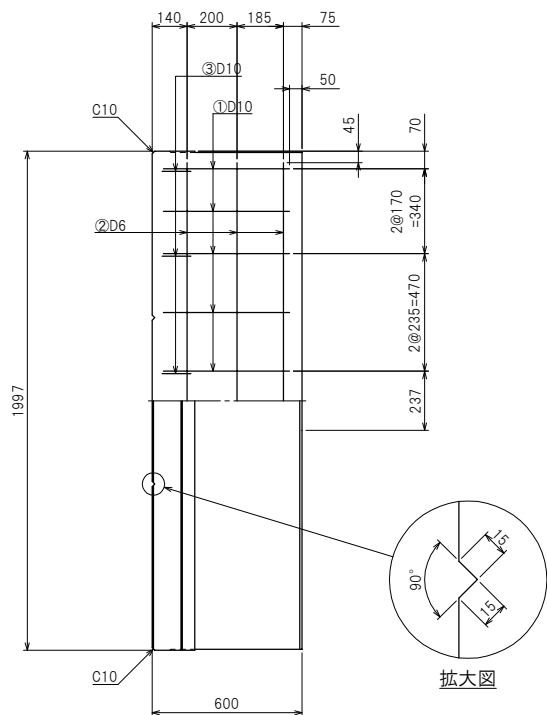
底板配筋図
