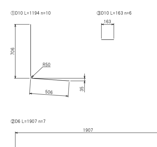
鉄筋加工図
