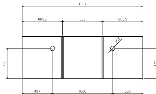
正面構造図
