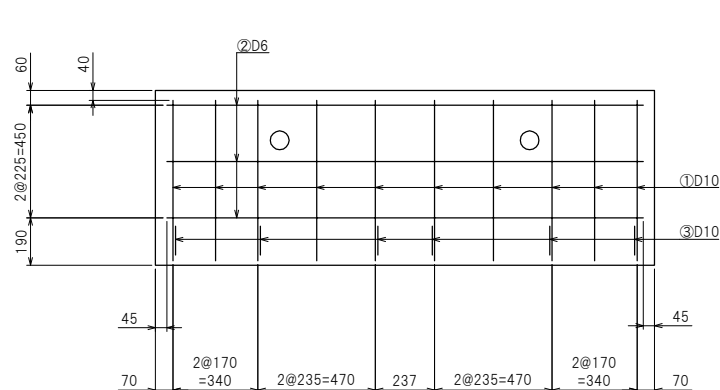
たて壁配筋図
