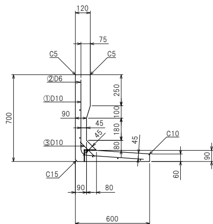
側面構造図
