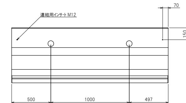
背面構造図
