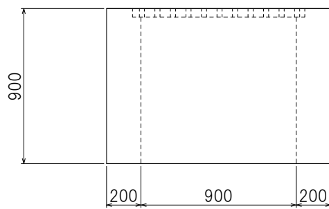
<側面図(短辺側)>
