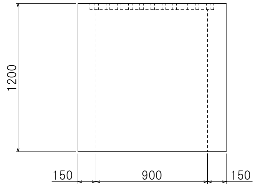
<側面図(短辺側)>
