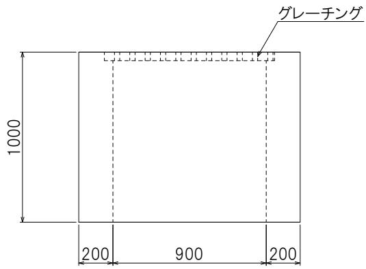
<側面図(長辺側)>
