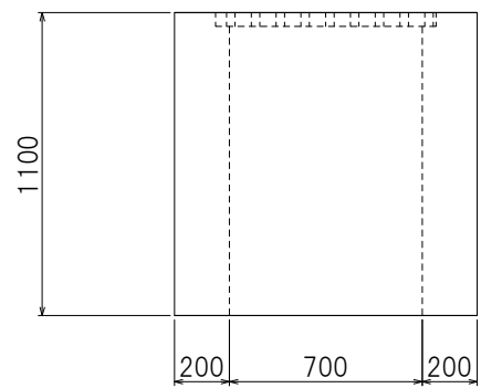
<側面図(短辺側)>
