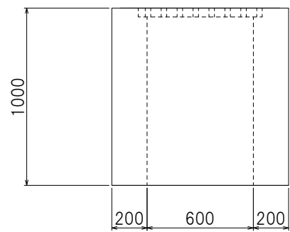
<側面図(短辺側)>
