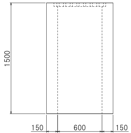
<側面図(短辺側)>
