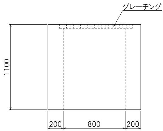
<側面図(長辺側)>
