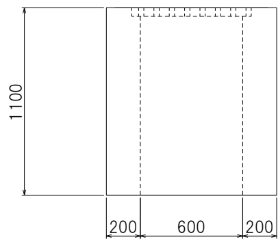
<側面図(短辺側)>
