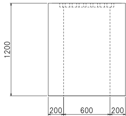
<側面図(短辺側)>
