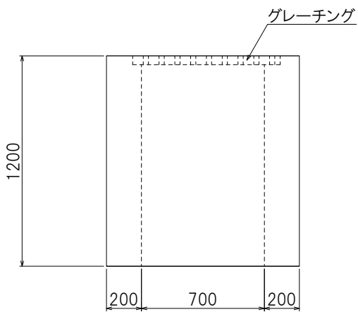
<側面図(長辺側)>
