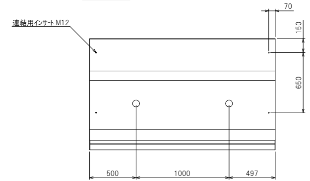
背面構造図
