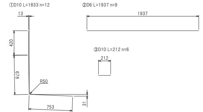
鉄筋加工図
