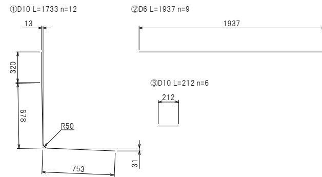
鉄筋加工図
