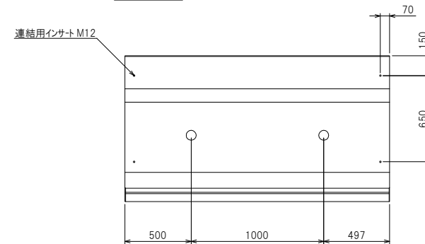
背面構造図
