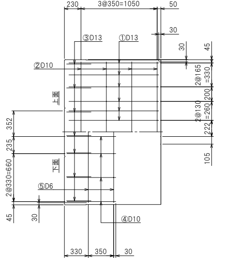
底板配筋図
