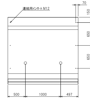
背面構造図
