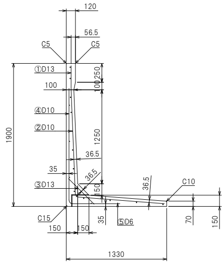
側面配筋図
