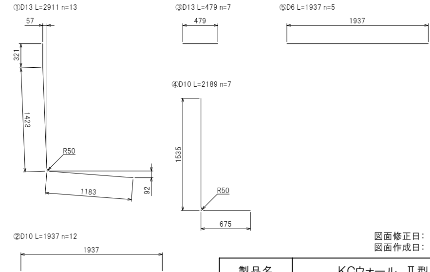
鉄筋加工図
