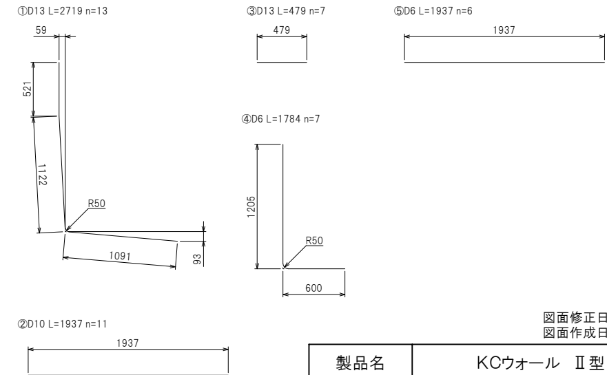
鉄筋加工図
