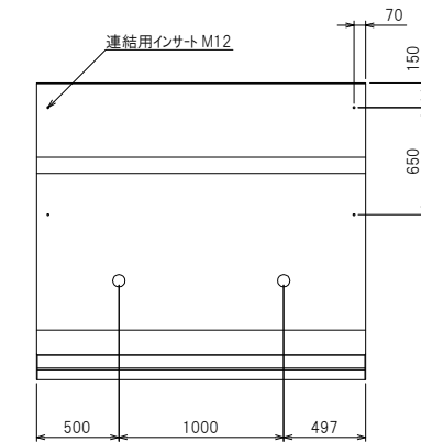
背面構造図
