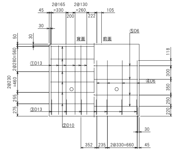
たて壁配筋図
