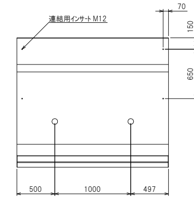
背面構造図
