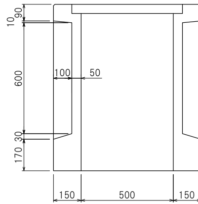
A-A断面図
