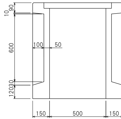
A-A断面図
