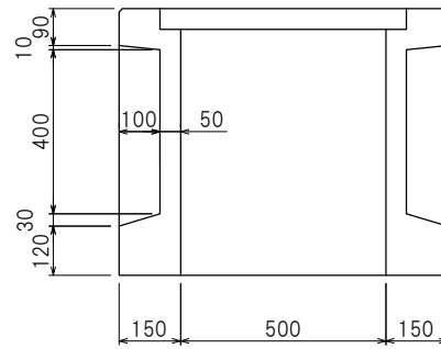
A-A断面図
