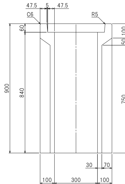
断面図
