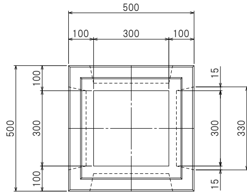
平面図(上側)
