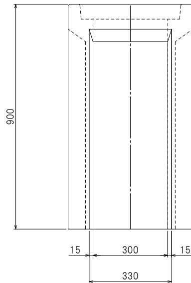
側面図
