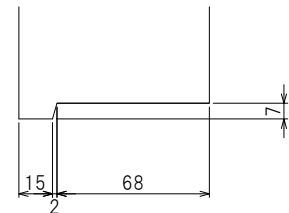
下部断面図
