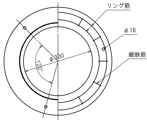
平面配筋図
