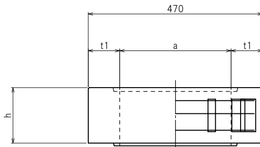
正面配筋図
