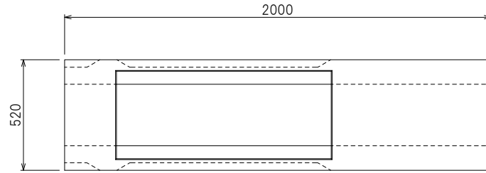
平面図
