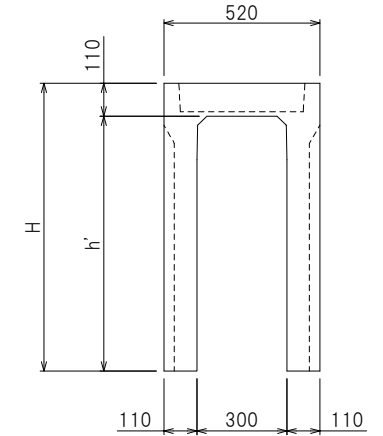
右側面図
