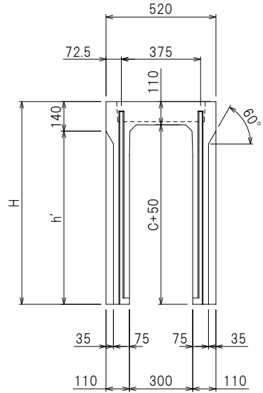
左側面図
