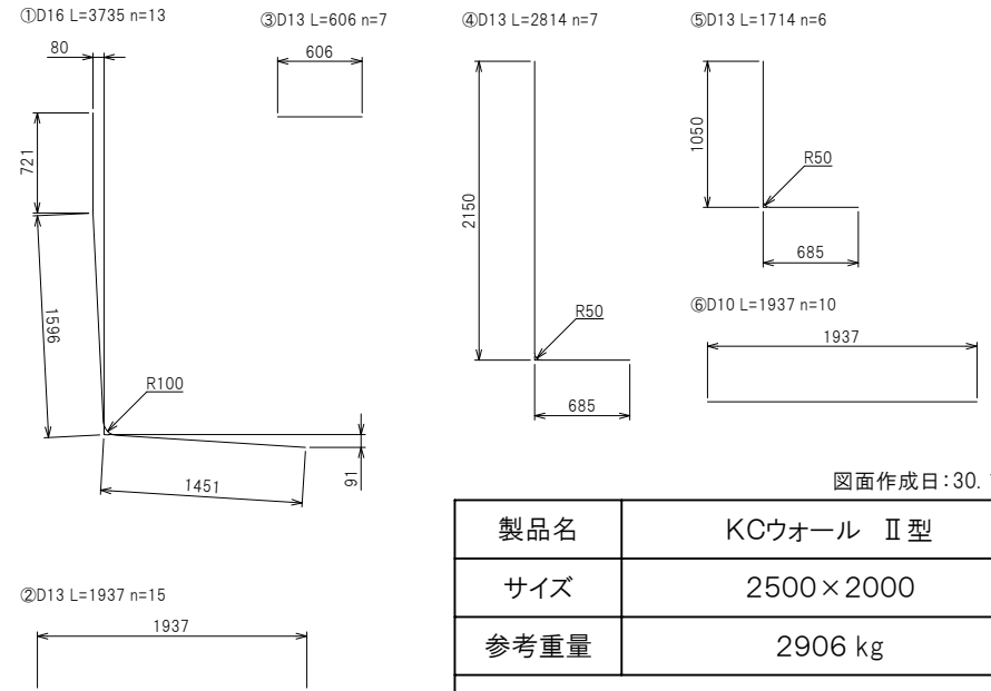
鉄筋加工図
