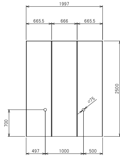
正面構造図
