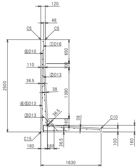
側面配筋図
