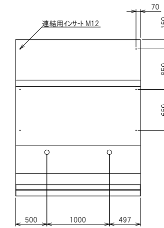
背面構造図
