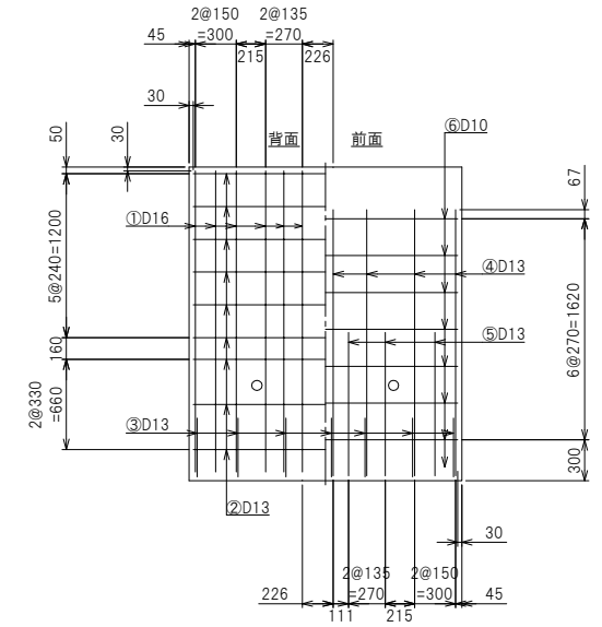
たて壁配筋図
