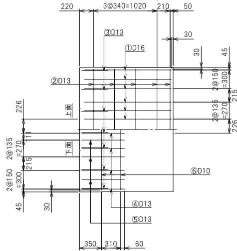
底板配筋図
