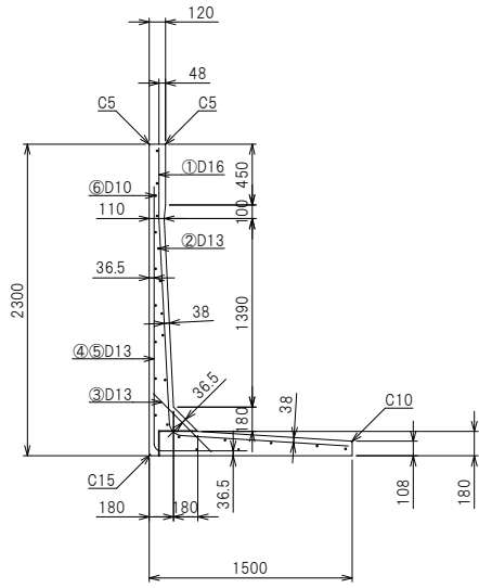
側面配筋図
