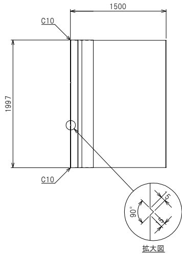
平面構造図
