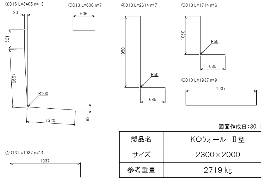
鉄筋加工図
