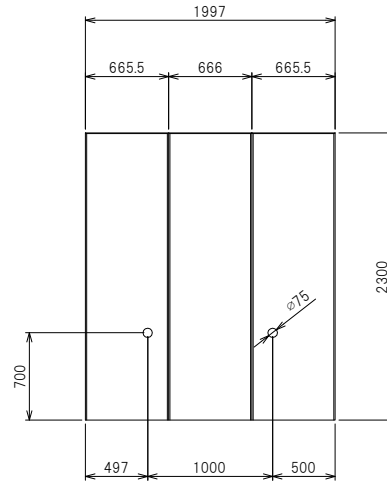
正面構造図
