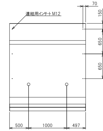
背面構造図
