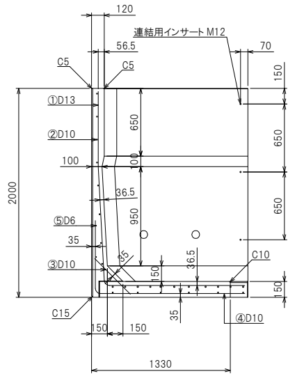
断面配筋図
