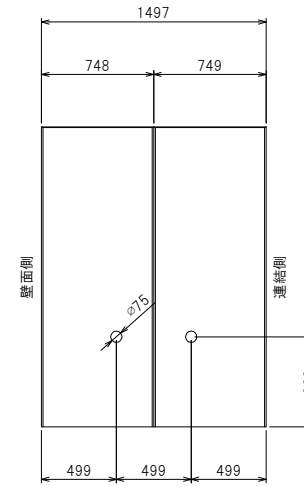
正面構造図
