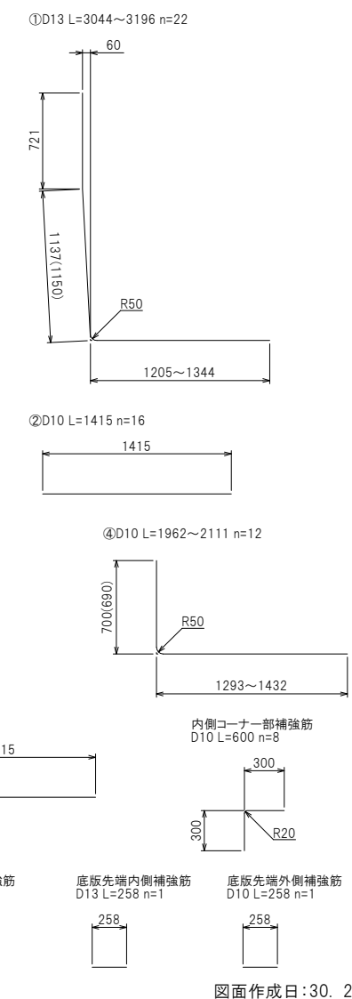
鉄筋加工図
