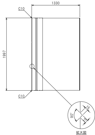
平面構造図
