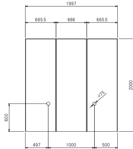
正面構造図
