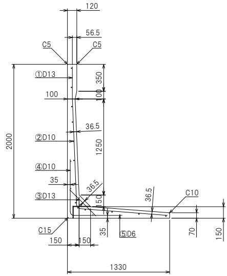
側面配筋図
