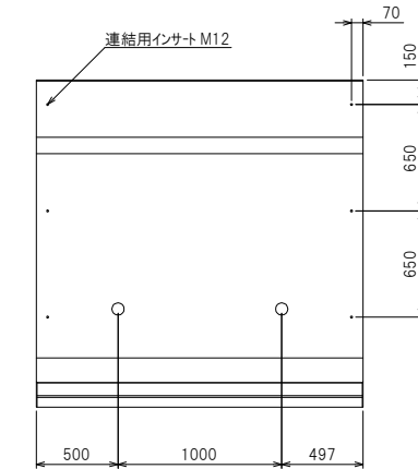
背面構造図
