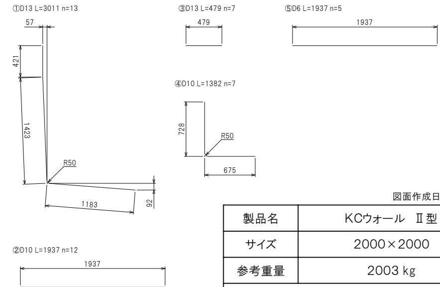
鉄筋加工図
