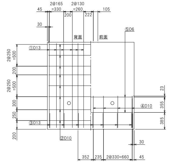
たて壁配筋図
