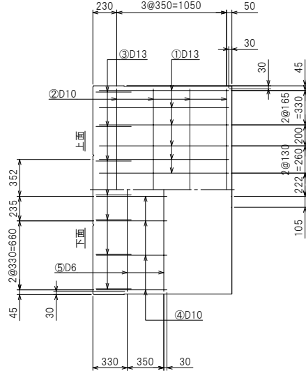
底板配筋図
