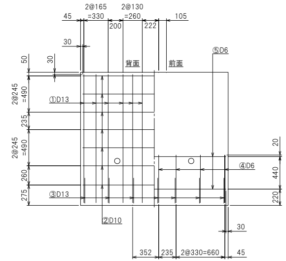
たて壁配筋図
