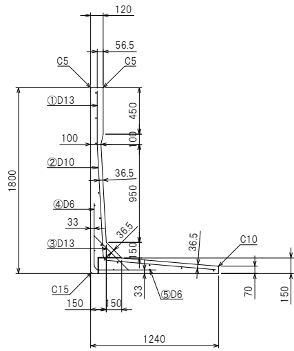
側面配筋図
