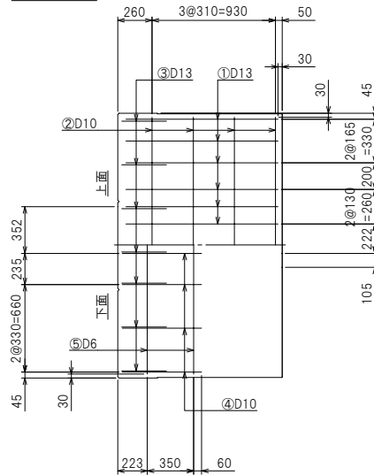
底板配筋図
