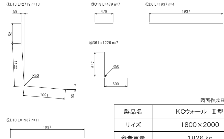
鉄筋加工図
